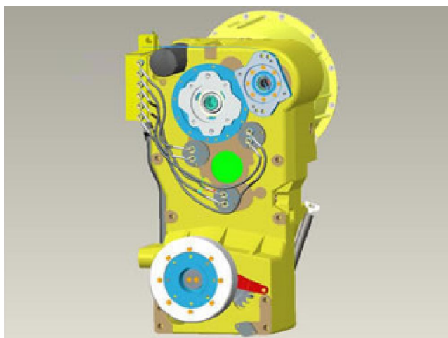
Гидравлическая коробка передач с электроуправлением BED4318
